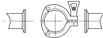
CLAMP FITTINGS BS 4825 - ISO 2852 - DIN 32676
